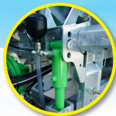
Гидроподвеска дышла
