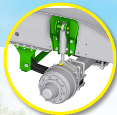
Направляющая ось и гидравлическая подвеска Hydro-Tandem
